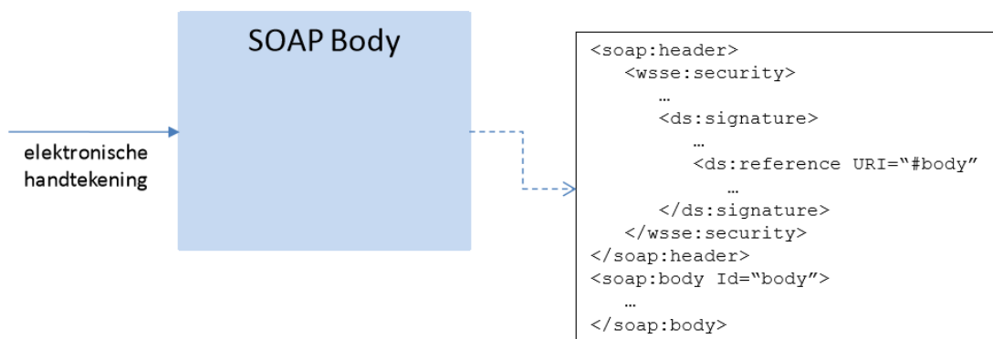
Figuur 3: SOAP-bericht met ondertekening
